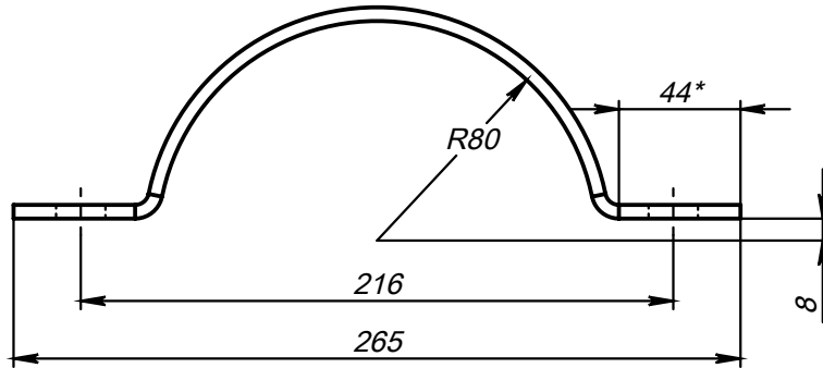
Поз.10 (Полухомут)
