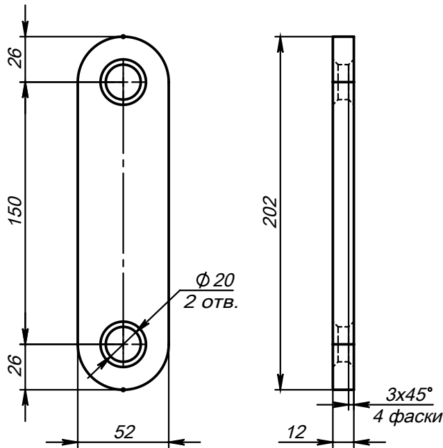
Поз.9 (Серьга)
