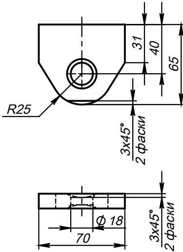
Поз.1 (Проушина)
