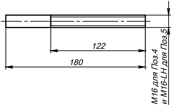
Поз.4 и Поз.5 (Шпилька)
