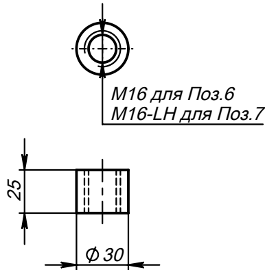
Поз.6 и Поз.7 (Гайка)
