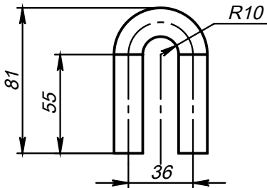
Поз.2 (Ушко)
